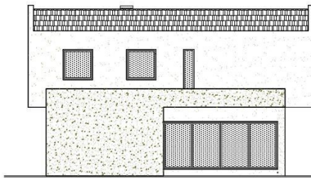
SJEVEROZAPADNO PROCELJE
