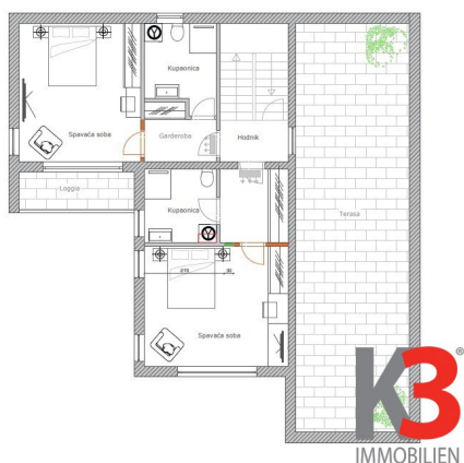
DISPOZICIJA NAMJEŠTAJA - KUĆA A - prizemlje M3 1:100
